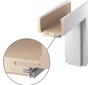
SOLID DIN DUO wykonana z wysokiej jakości drewna klejonego warstwowo (część zasadnicza), opaski wykonane z wysokiej jakości MDF
